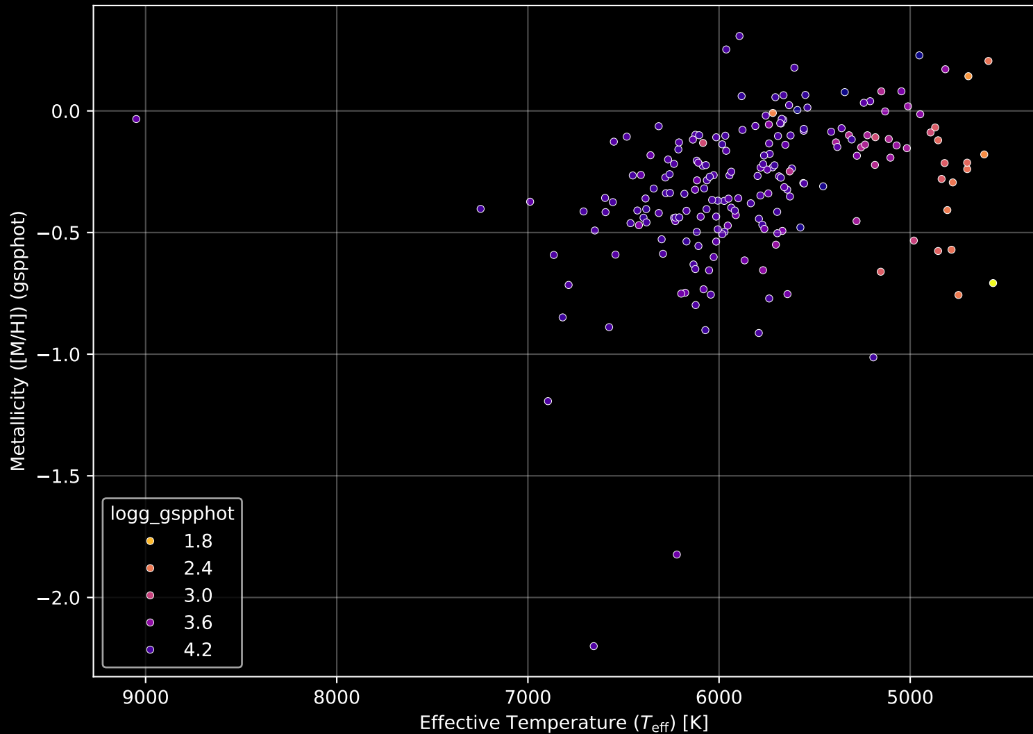
GALAH DR4 Field: [659] Stellar Population Parameters (n= 201)
